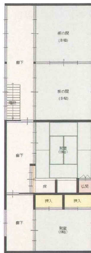
＜門屋 2階＞
