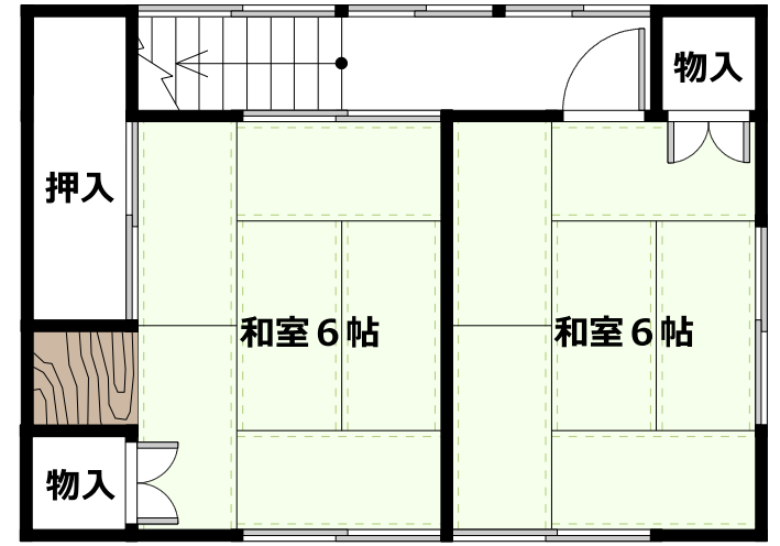
< 2階 >
