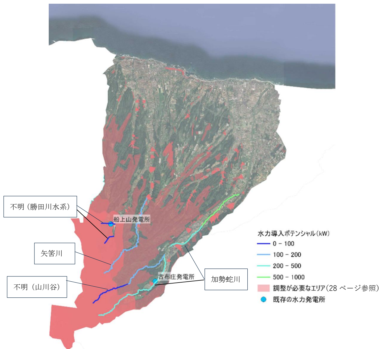
図31. 小水力発電の導入ポテンシャルマップ
