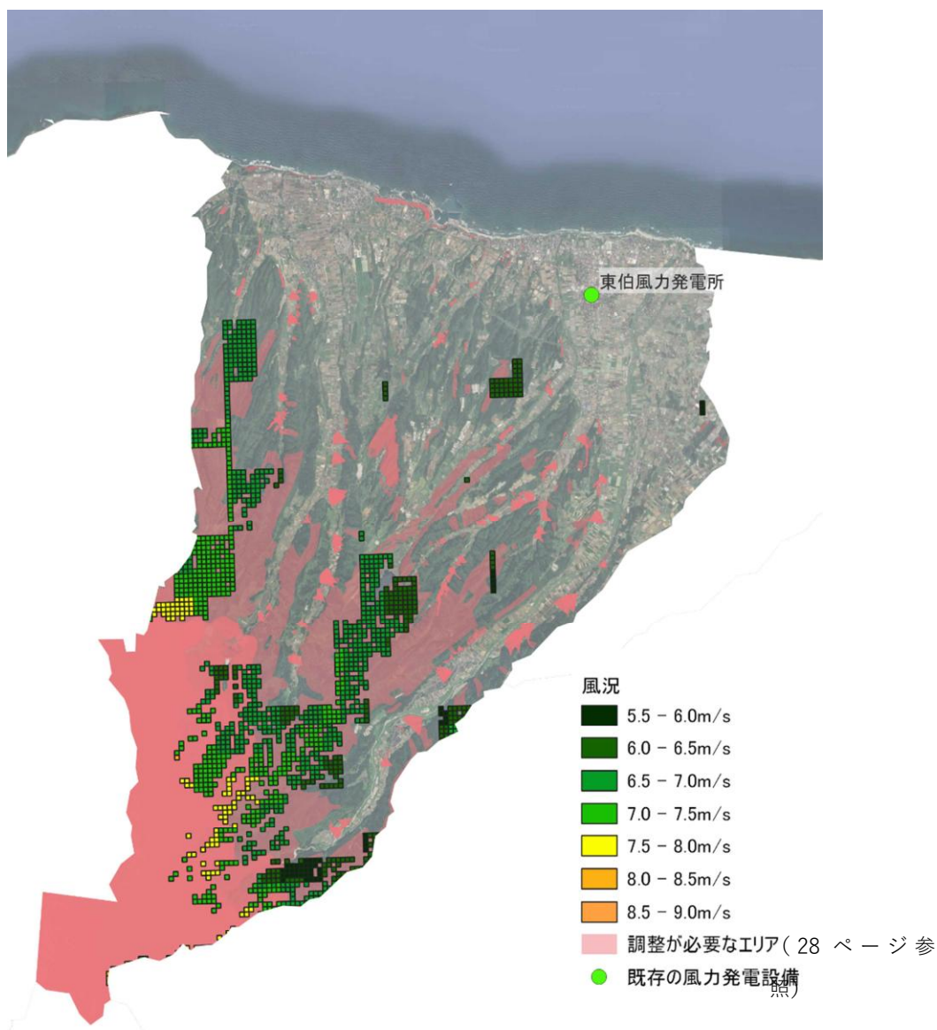
図33. 風力発電の導入ポテンシャルマップ
