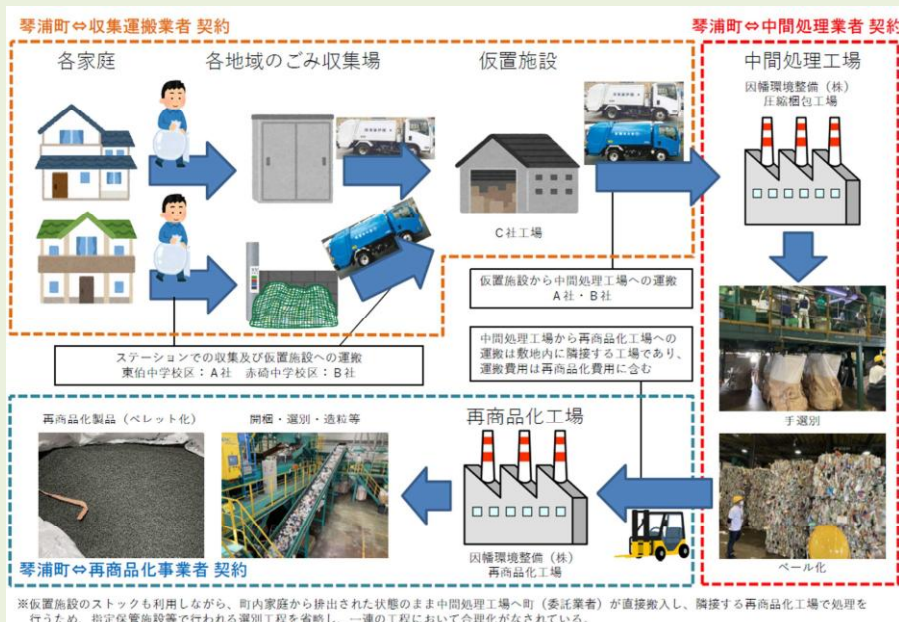
図53. 琴浦町プラスチック一括回収及び再商品化に係る工程
