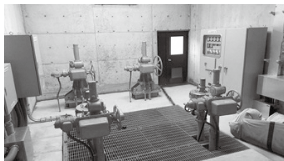
船上山ダム放流設備操作盤の更新
