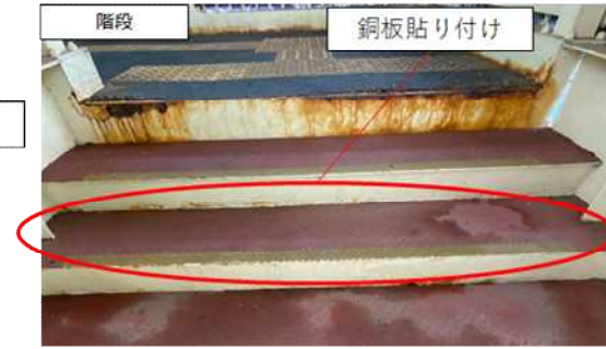
劣化程度：5（銅板貼り付け前） 状態：元の板に穴が開いているため、編銅板を貼り付け
