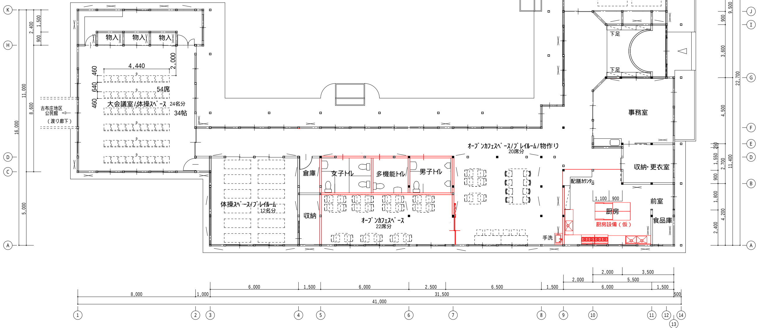
旧古布庄保育園 平面図 S=1:150 延床面積：452.850m 2
