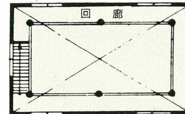
2階吹抜平面図
