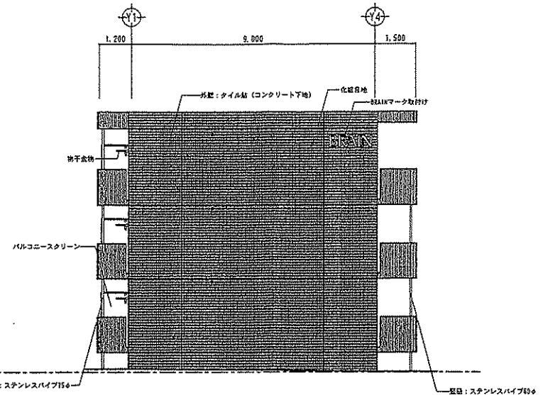
東立面图 SCALE = 1:100
