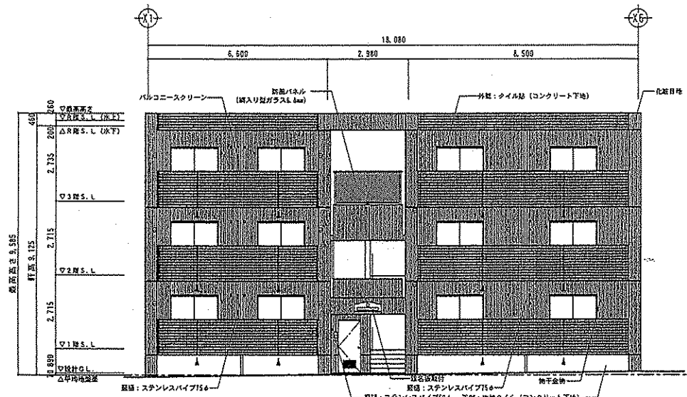
南立面图 SCALE = 1:100
