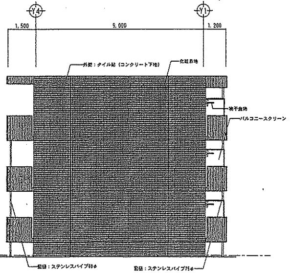
西立面图 SCALE = 1:100
