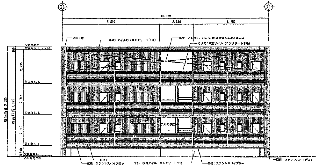
北立面图 SCALE = 1:100
